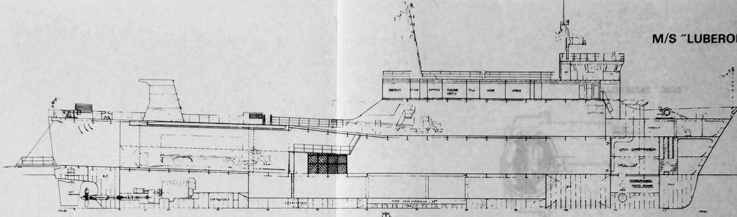
- PONT SUPERIEUR -
